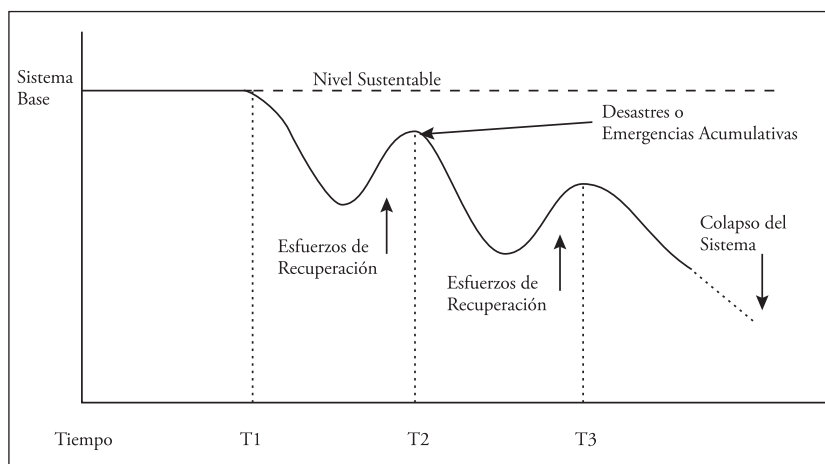
Gráfico 1 Entropía puntuada
